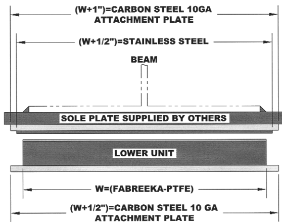
END ELEVATION
